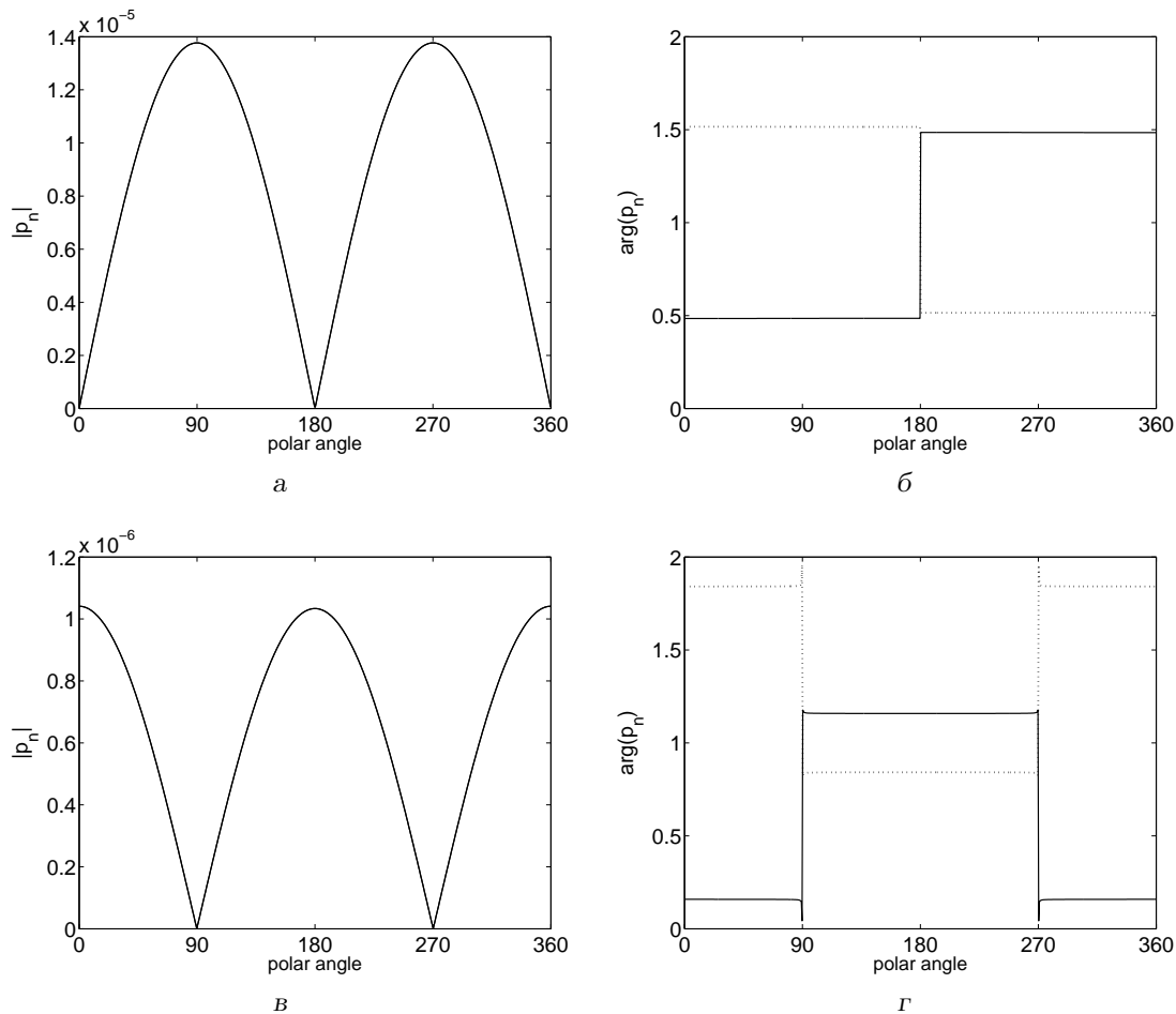
Рис. 9. Модули и фазы первых двух гармоник давления p_n на расстоянии 1 м от центра цилиндра ( Re=200 ): а - |p_n| при n=\pm 1 , б - \arg(p_n) при n=\pm 1 , в - |p_n| при n=\pm 2 , г - \arg(p_n) при n=\pm 2 ; б, г - сплошные - n=1, 2 , штриховые - n=-1, -2 (единица по вертикальной оси соответствует \pi рад)
