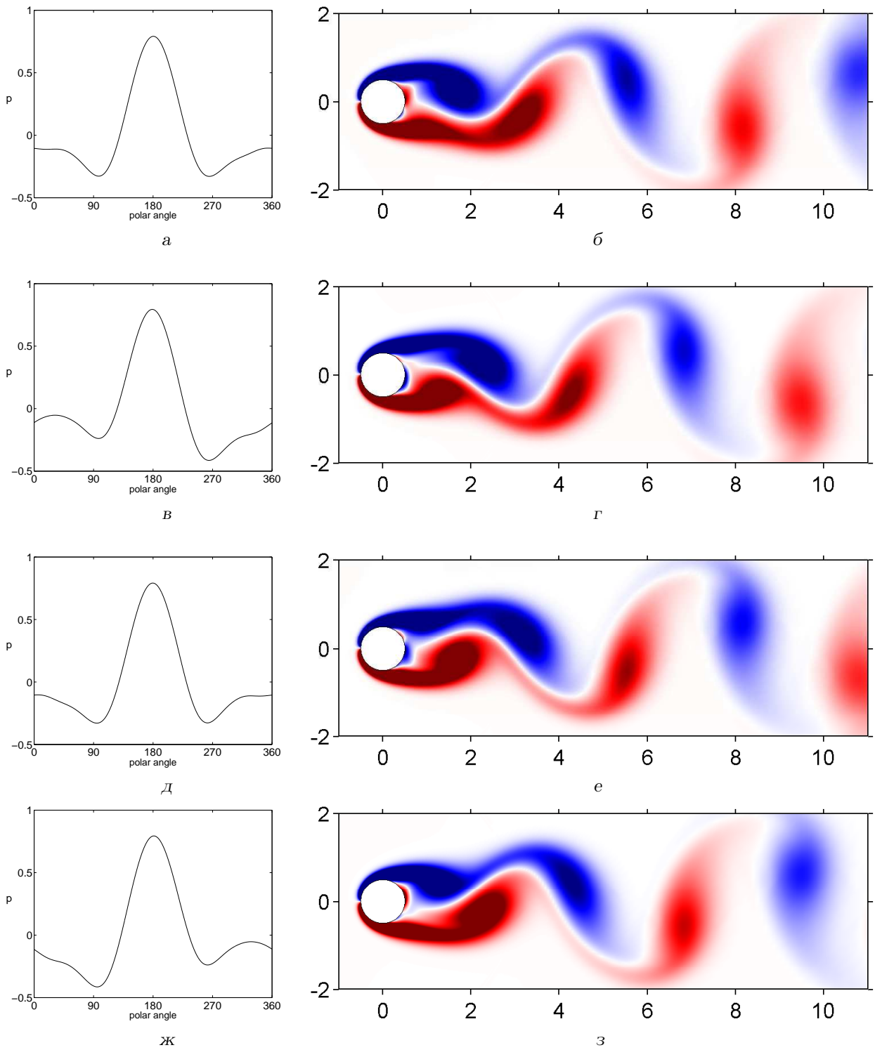
Рис. 3. Течення при Re=100 в різні моменти часу (в лівій колонці – розподіл тиску на поверхні циліндра, а в правій – поле завихреності): а, б - t=0 , в, г - t=T/4 , д, е - t=T/2 , ж, з - t=3T/4
