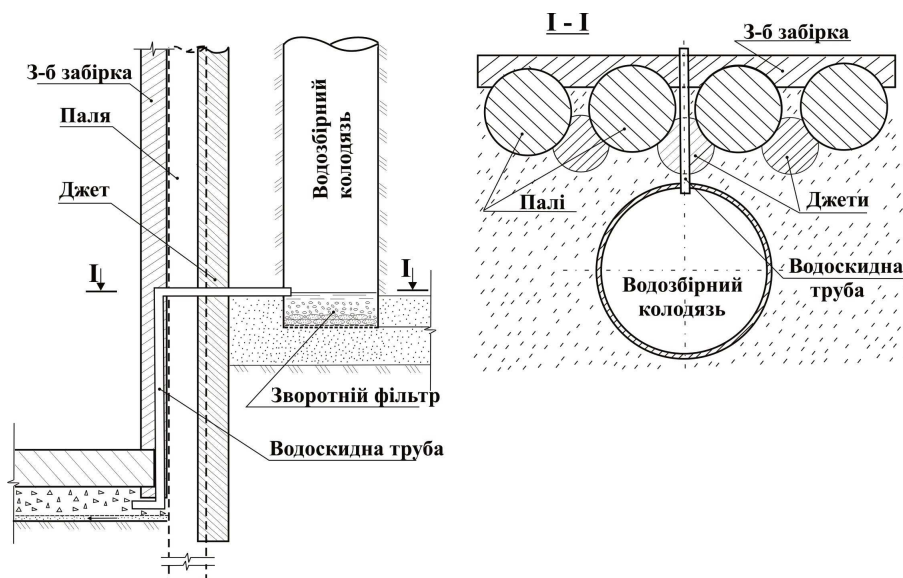
Рис. 9. Конструктивні елементи дренажу з водозбірних колодезів в поєднанні з пластовим дренажем для зняття баражного ефекту
