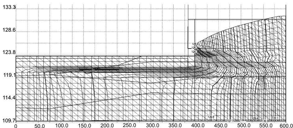
Рис. 6. Положення еквіпотенціалей і кривої депресії по розрізі I-I при улаштуванні дренажу за рекомендованою схемою
