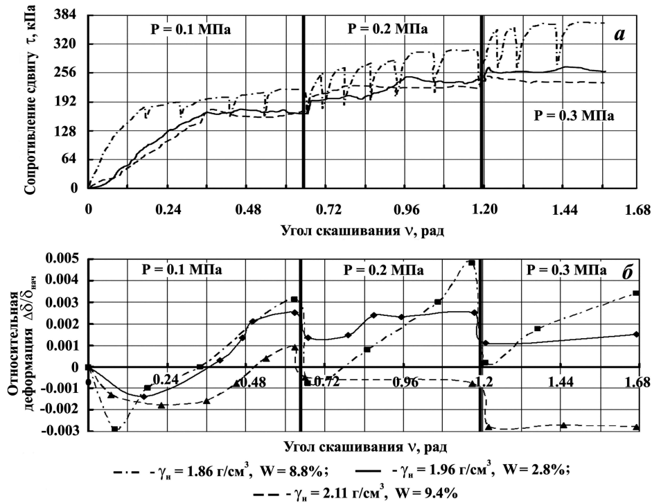
Рис. 7. Результаты исследований на сдвиг крупнозернистого песка: а – усилие сдвига – угол скашивания; б – относительная деформация осадки – угол скашивания
