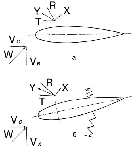
Рис. 1. Силы, действующие на крыло: а – крыло с жесткой заделкой, б – крыло с упругой заделкой
