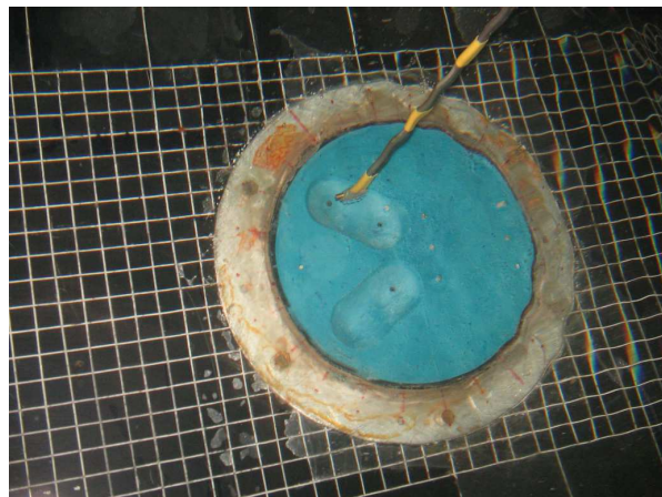
Рис. 6. Розташування датчиків динамічного тиску над обтічною поверхнею овальної лунки
