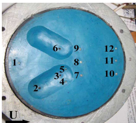
Рис. 4. Розташування датчиків пульсацій пристінного тиску на обтічній поверхні овальних лунк і пластини
